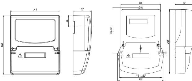
Рисунок А.1 – Тип корпуса Р32
