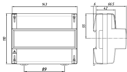
Рисунок А.3 – Тип корпуса Р31
